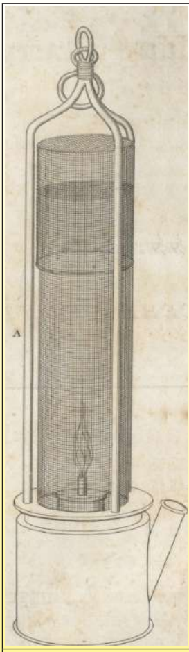
1815 La lampe de sécurité de mineur inventée par Humphry Davy
