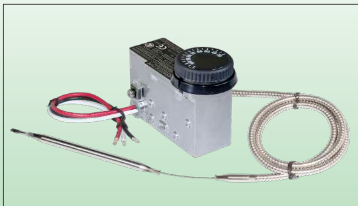
Thermostat KAA avec manette softgrip 66MZ et enjoliveur 66EN1
