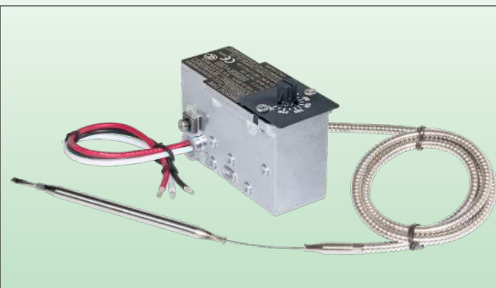
Thermostat KAA avec manette miniature 66MQ et cadran gradué 66CP02
